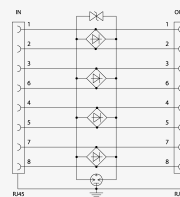
Schéma zapojenia
