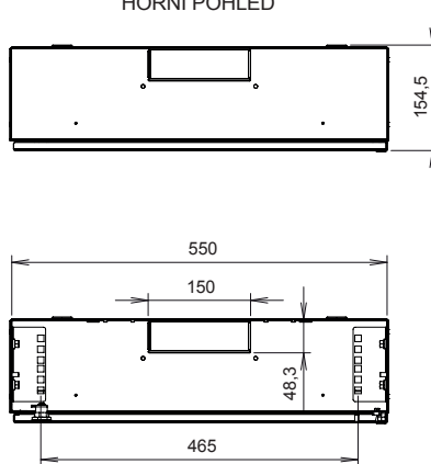
HORNÍ POHLED
