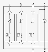
Schéma zapojenia
