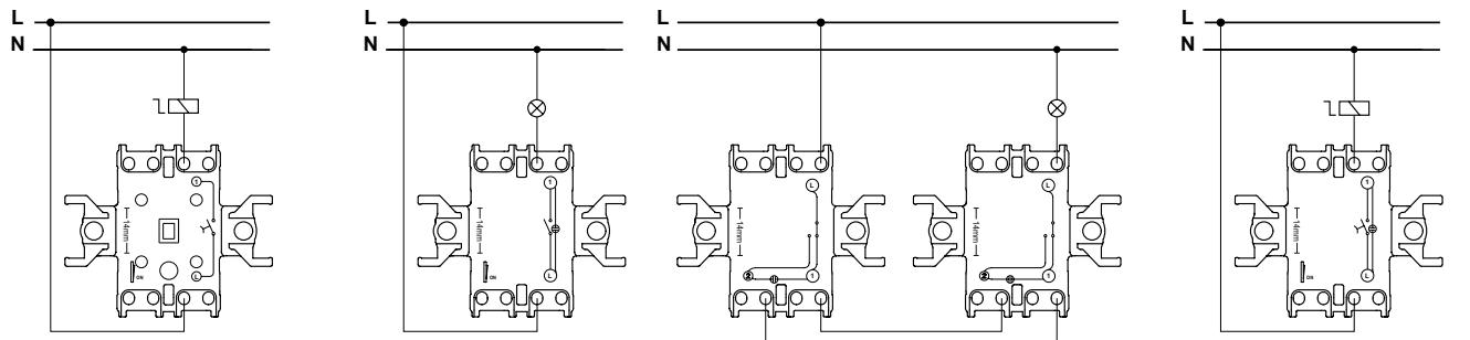
Tlačidlo
