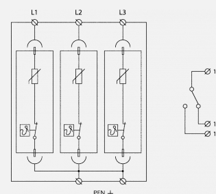
Schéma zapojenia
