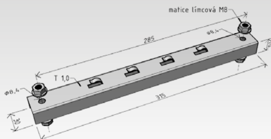
podpěra PZM 250
