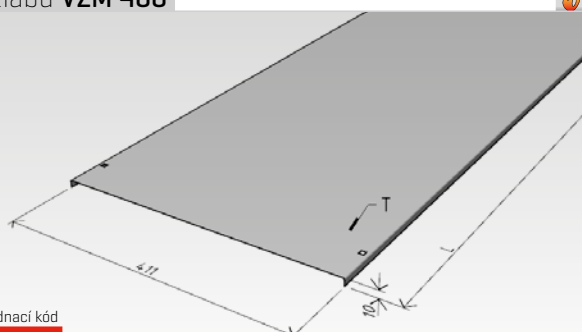
víko žlabu VZM 400
