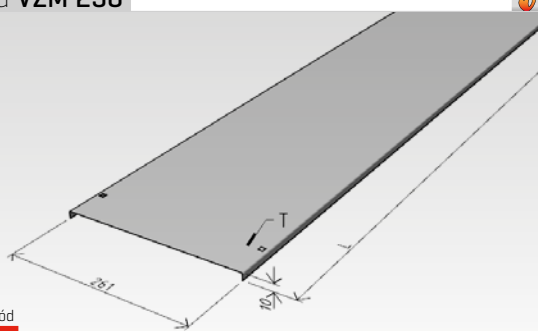
víko žlabu VZM 250
