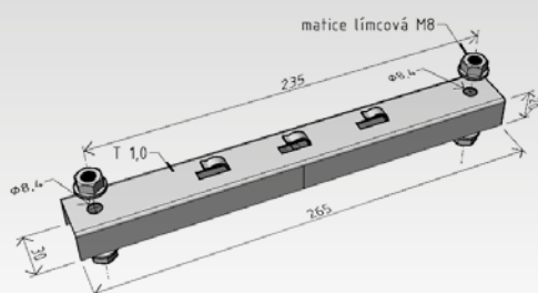
podpěra PZM 200
