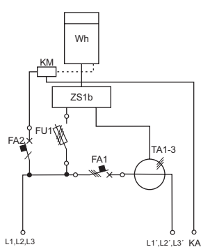
Zpojenie SSD
