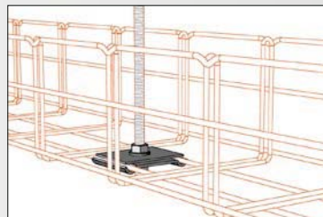
ukázka montáže
